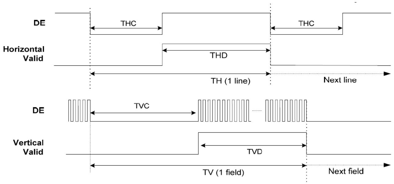
DE Mode Input Timing
