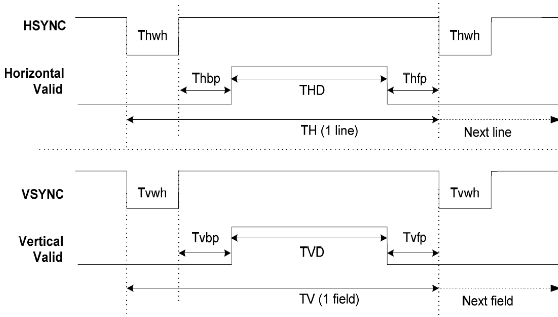
HV Mode Input Timing
